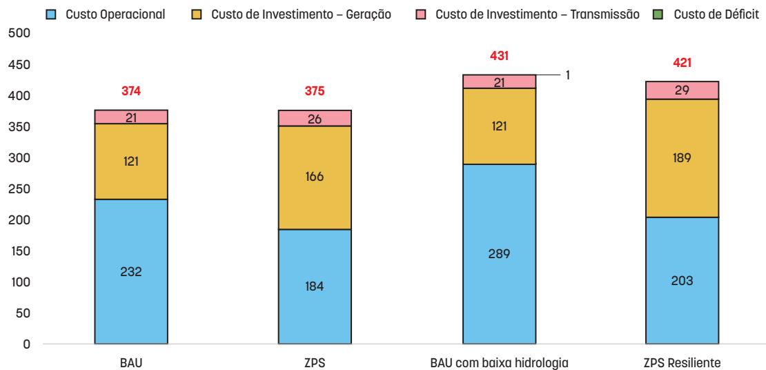
FIGURA 16. Custo líquido presente do sistema elétrico brasileiro em 2050, em diferentes cenários (R$ bilhão)
